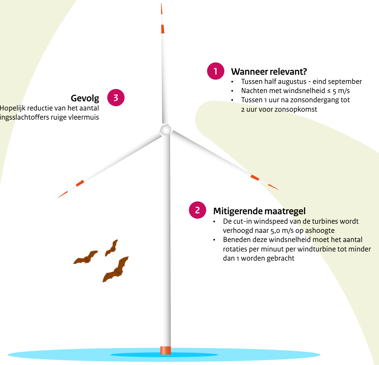
Figuur 7.5: Stilstandvoorziening voor vleermuizen beschreven in het Kavelbesluit voor windenergiegebied Borssele WETTENBANK .
