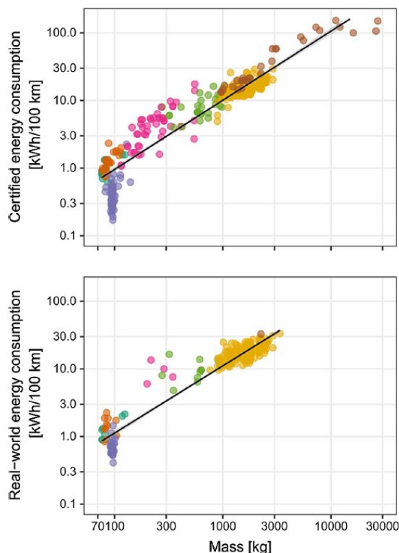
Figuur 2.7 Energiegebruik naar massa elektrische voertuigen op een log-log-schaal
