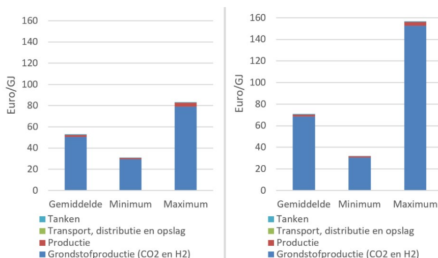
Figuur 4.10 Overzicht van de kosten van methanol voor de maritieme sector, links gebaseerd op CO 2 -afvang bij industriële puntbronnen (CC) en rechts op CO 2 -afvang uit de lucht (DAC)
