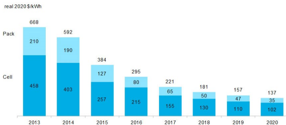
Figuur 2.8 Ontwikkeling van batterij- en accuprijzen per kWh
