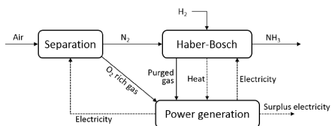
Figuur 4.3 Schematisch overzicht van N 2 productie en ammoniak productie in een geïntegreerd systeem
